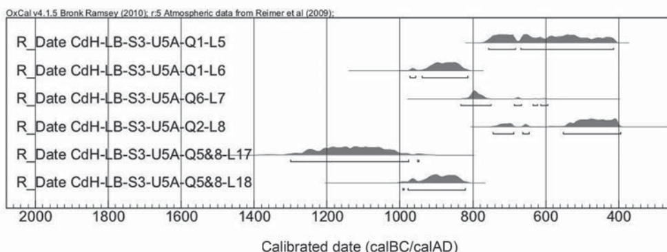
Fig. 19. Fechados de una sola unidad de excavación (U5A) de La Banda, de los trabajos de John Wolf. Se ordenan, estratigráficamente, desde la capa 18 hasta la capa 5 (elaboración del gráfico: John W. Rick, por medio del programa OxCal v4.1.5 [Bronk Ramsey 2010]).
