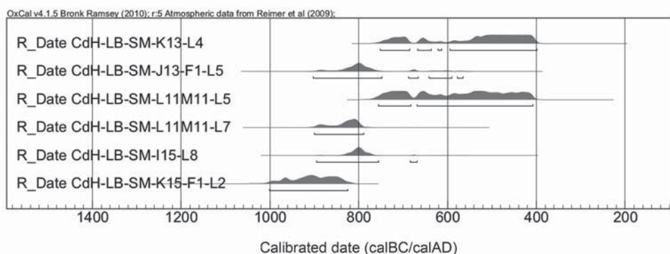
Fig. 20. Fechados de la zona La Banda SM, excavaciones de Matthew Sayre. Se ordenan, estratigráficamente, desde la capa 8 hasta la capa 4; el fechado F1-L2 corresponde a un elemento estratigráficamente inferior a la capa 8 (elaboración del gráfico: John W. Rick, por medio del programa OxCal v4.1.5 [Bronk Ramsey 2010]).
