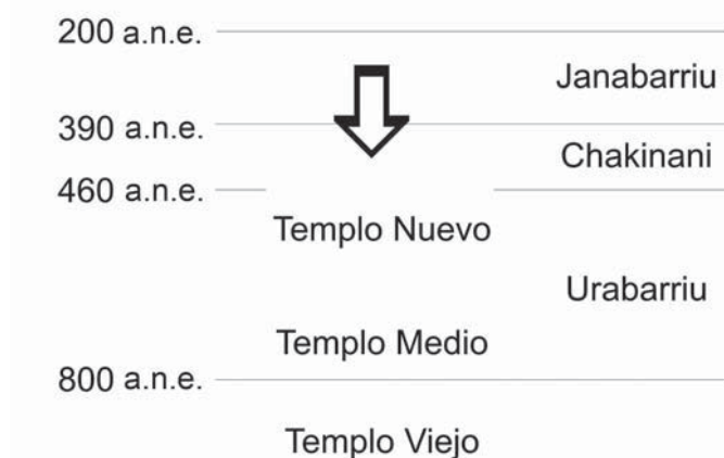
Fig. 24. El errado modelo «deslizado», en el que, por tratar de acomodar nuevas fechas relativamente tempranas para la arquitectura de Chavín, los miembros del Proyecto de Investigación y Conservación de Chavín de Huántar desligaron las fases arquitectónicas de las fases cerámicas, con lo que se hizo retroceder la arquitectura hacia el pasado (elaboración del gráfico: John W. Rick).
