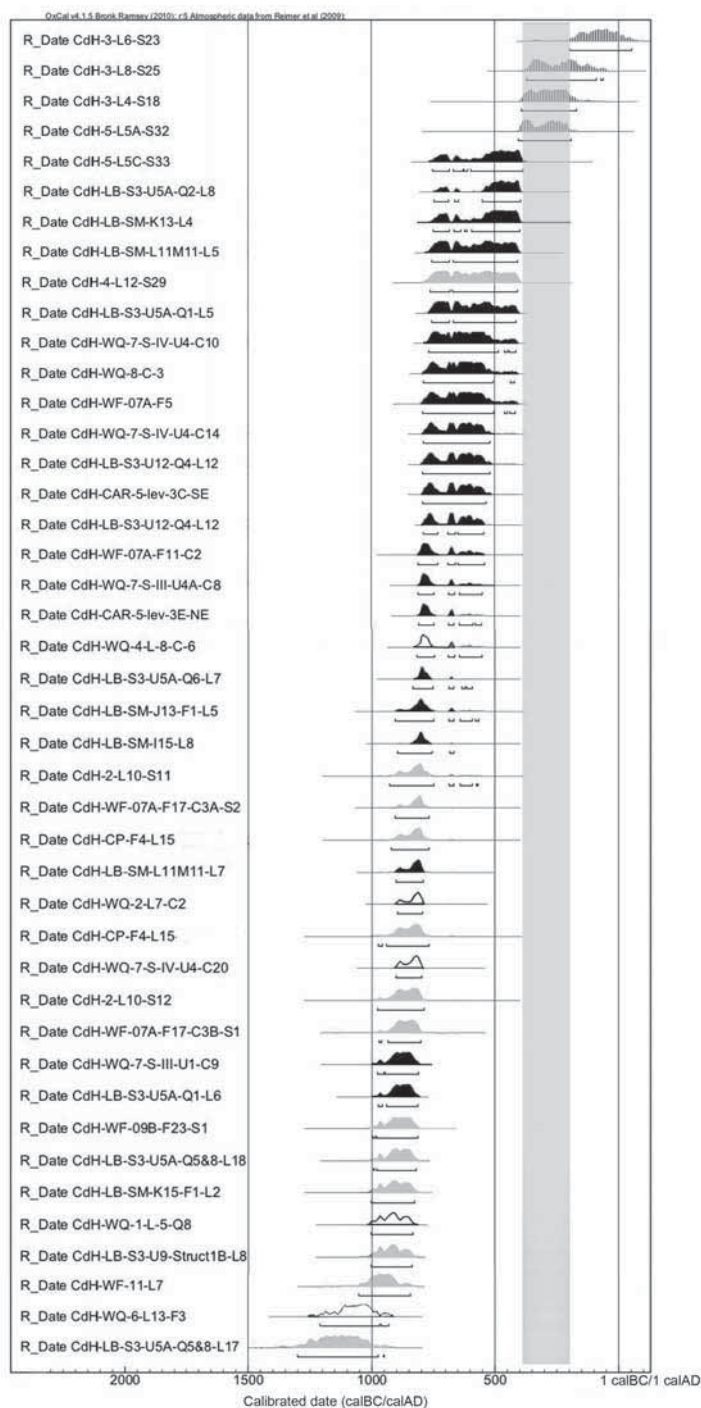
Fig. 21. Gráfico de todos los fechados usados en este artículo pertenecientes a las excavaciones del Proyecto Chavín. La banda vertical gris indica la temporada propuesta por Burger para su fase Janabarriu. Los fechados con curvas de líneas verticales provienen de contextos con cerámica huaraz; los de curvas de color negro corresponden a contextos con cerámica janabarroide; los de curvas de color gris tienen muestras insuficientes para determinar su cerámica y los de curvas con una línea de contorno pero blanco en su interior tienen cerámica suficiente, pero faltan evidencias de que sean de carácter janabarroide (elaboración del gráfico: John W. Rick, por medio del programa OxCal v4.1.5 [Bronk Ramsey 2010]).
