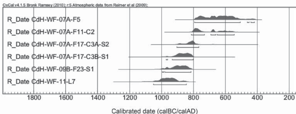
Fig. 17. Fechados de contextos chavín del Campo Oeste. WF-07A indica el contexto de una estructura de estilo Mito (véase Contreras 2010); los otros contextos son de distintas unidades de excavación del Campo Oeste (elaboración del gráfico: John W. Rick, por medio del programa OxCal v4.1.5 [Bronk Ramsey 2010]).
