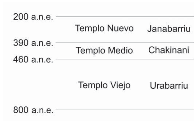
Fig. 23. Gráfico del modelo «coterminal», en que los tres supuestos periodos propuestos coinciden exactamente con los cambios en la cerámica y la arquitectura monumental en el sitio de Chavín de Huántar (elaboración del gráfico: John W. Rick).
