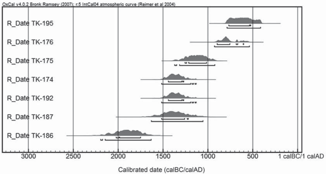
Fig. 9. Fechados de La Pampa. Las fechas TK-176 y TK-195 corresponden a la fase La Pampa, caracterizada por presentar rasgos cerámicos janabarroides. Nótese que los cuerpos centrales de los fechados se ubican entre 850 y 400 a.n.e. (elaboración del gráfico: Christian Mesia, por medio del programa OxCal v4.0.2 [Bronk Ramsey 2007]).
